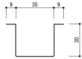
通し吊子
