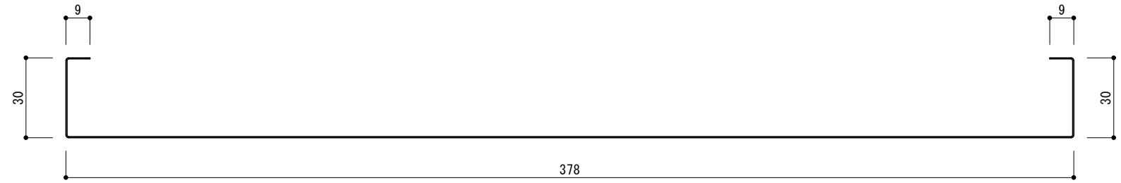
ドブ板
